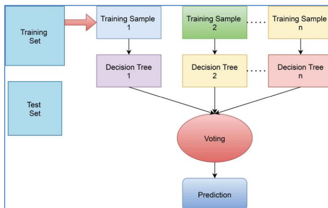
Hình 3. Lưu đồ thuật toán Random Forest [19]
