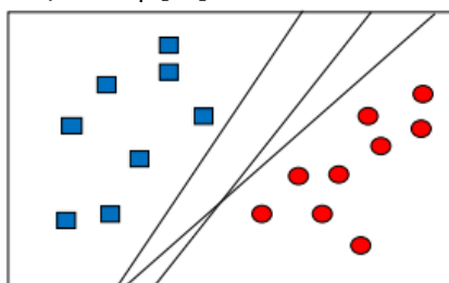
Hình 2. Có vô số đường thẳng phân tách hai lớp dữ liệu [18]
