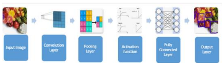
Hình 5. Kiến trúc CNN [22]
